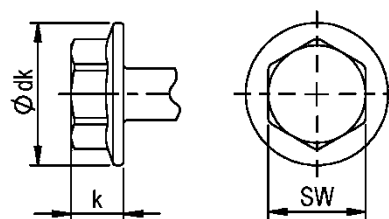
Sechskantkopf mit Bund
